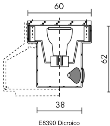
E8390 Dicroico
